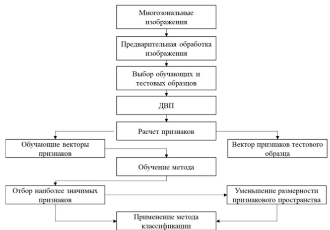
Рисунок 1 - Блок-схема предложенного метода интерпретации космических снимков
